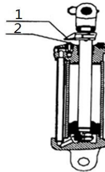
Рис. 5-11 Цилиндр в сборе.
