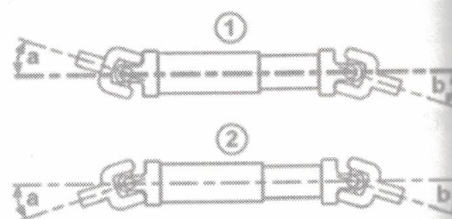
Складывание телескопической трансмиссии
