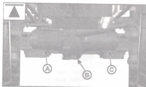
Рис. 5.23c. Поднятие передней части трактора
