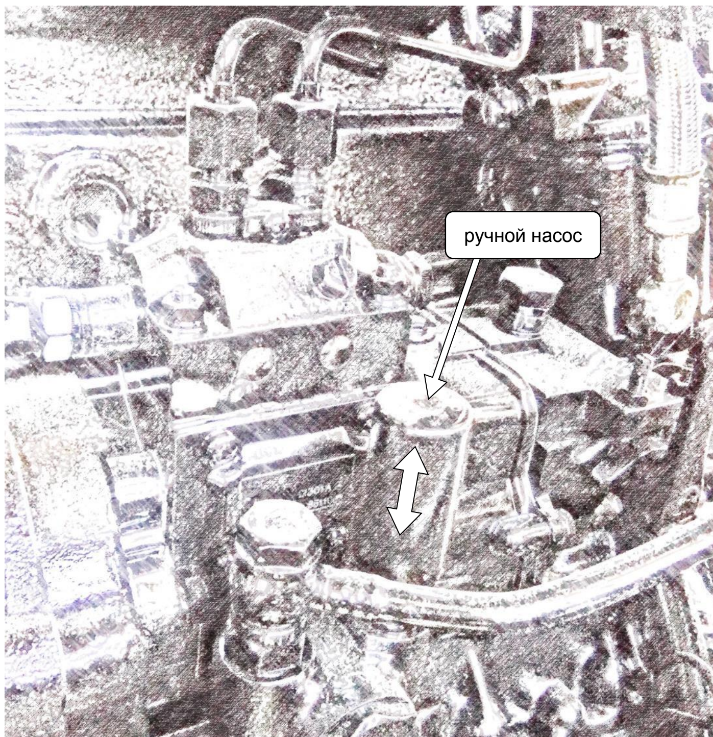
Рис. 3-1. Ручной насос
