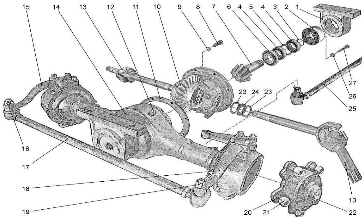
Рис. 8.1 Передний ведущий мост
