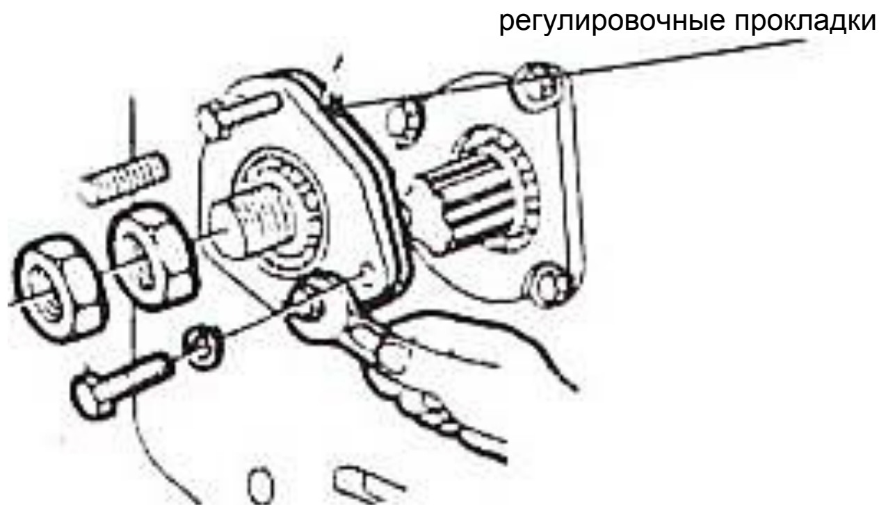
Рис. 5-5. Регулировка центральной передачи I
