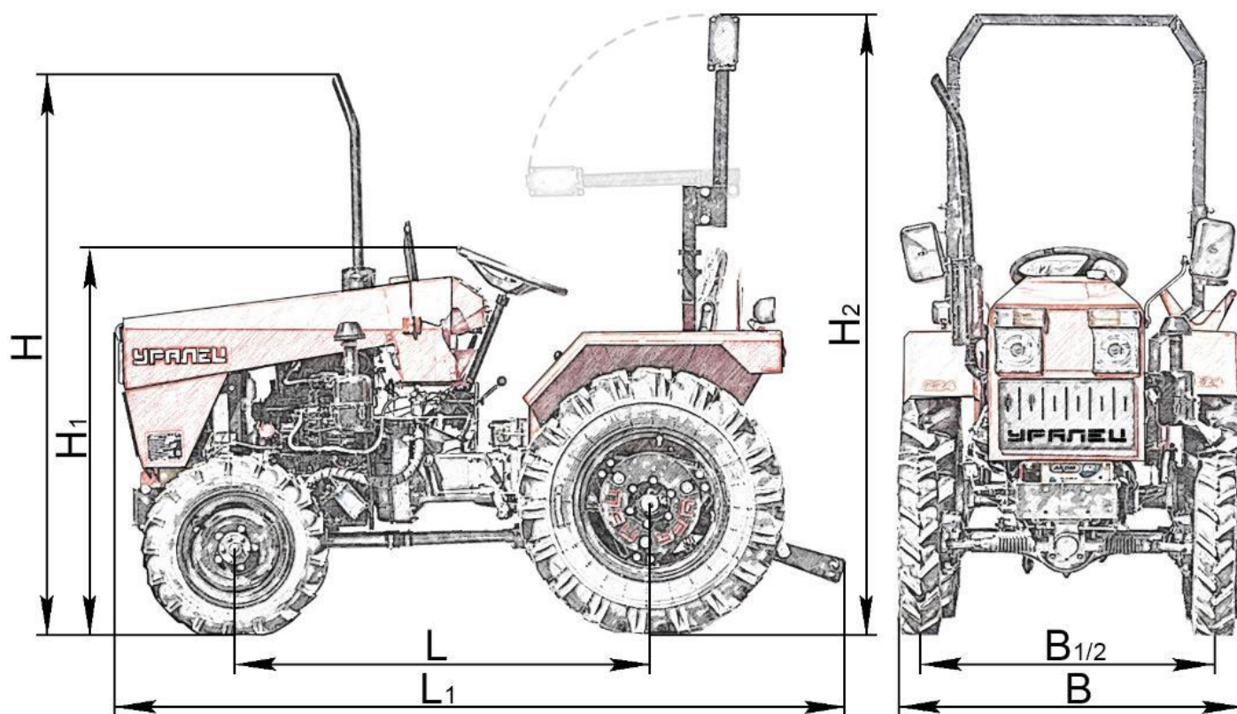
Рис. 1-1. Габаритные размеры трактора
