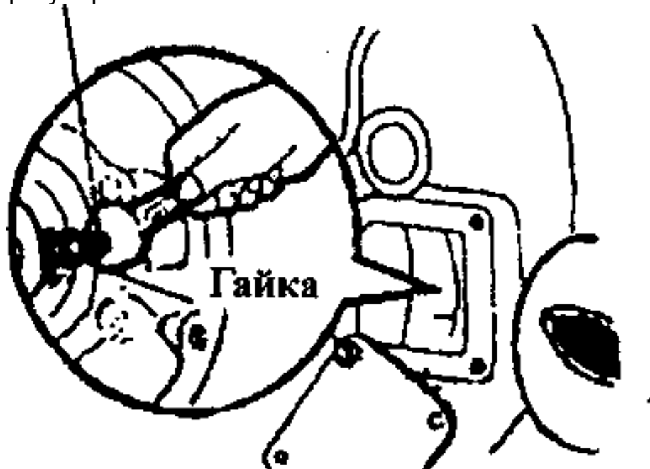
Рис. 5-2. Регулировка зазора между отжимным кольцом и выжимным подшипником
