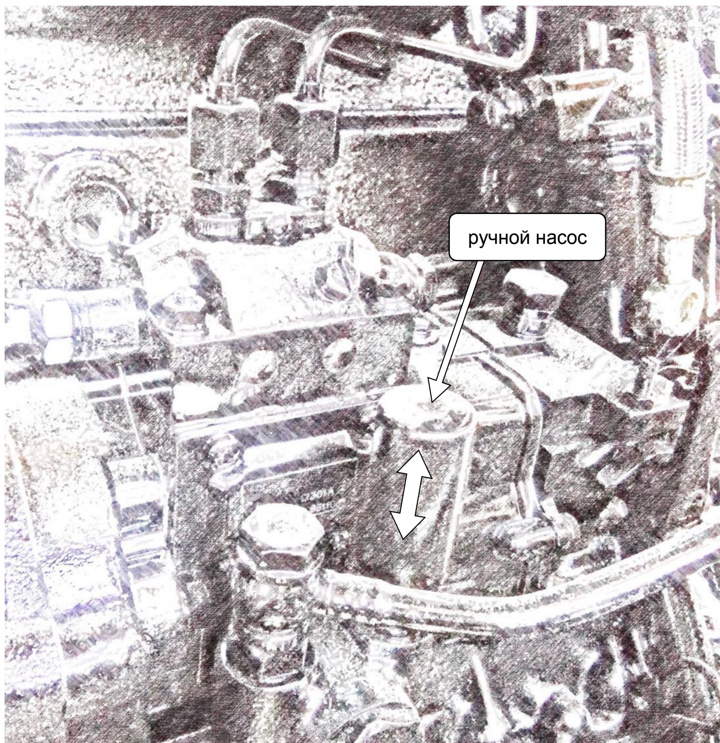
Рис. 3-1. Ручной насос
