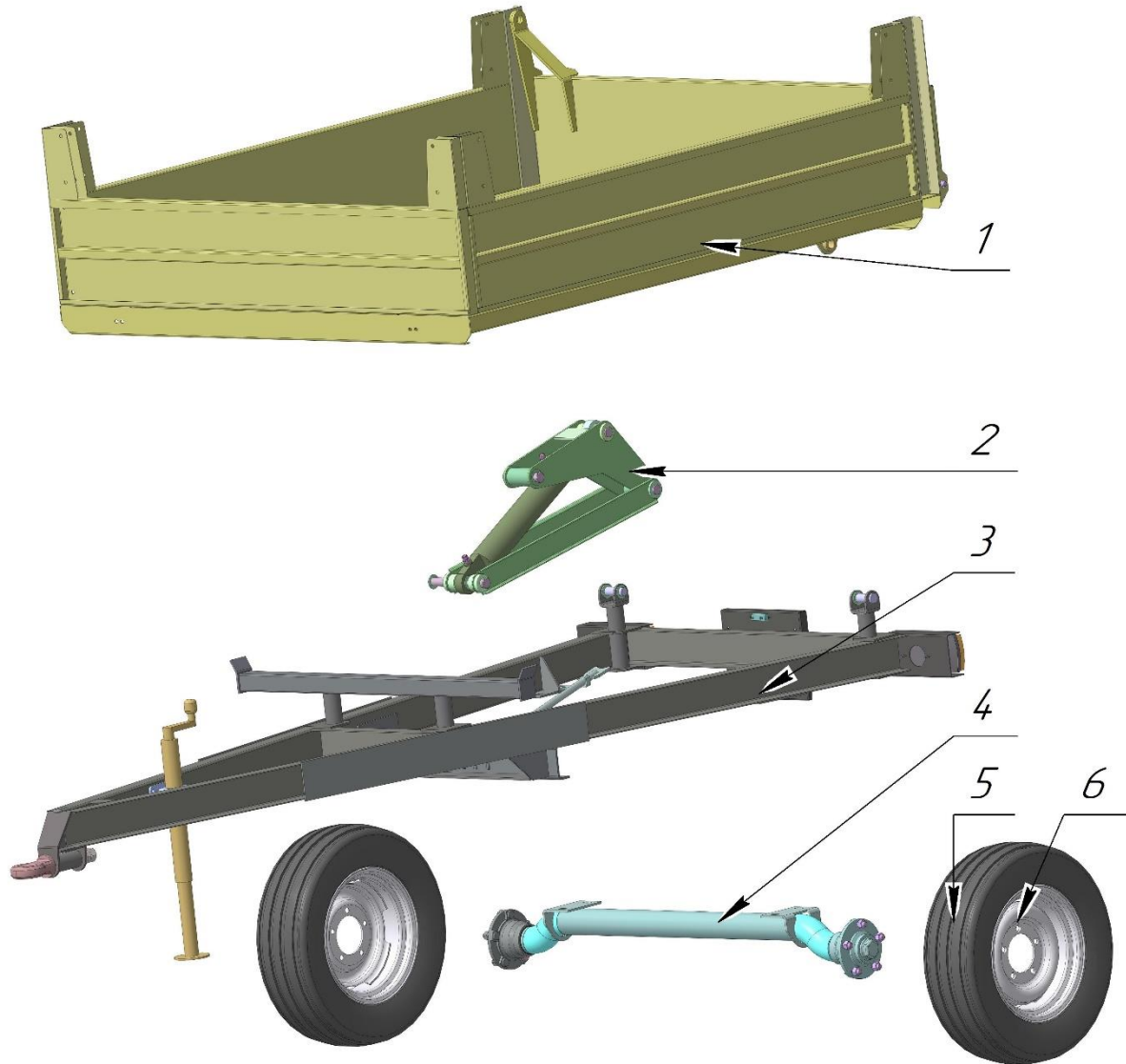
ПОЛУПРИЦЕП-САМОСВАЛ (Рис. 1)
