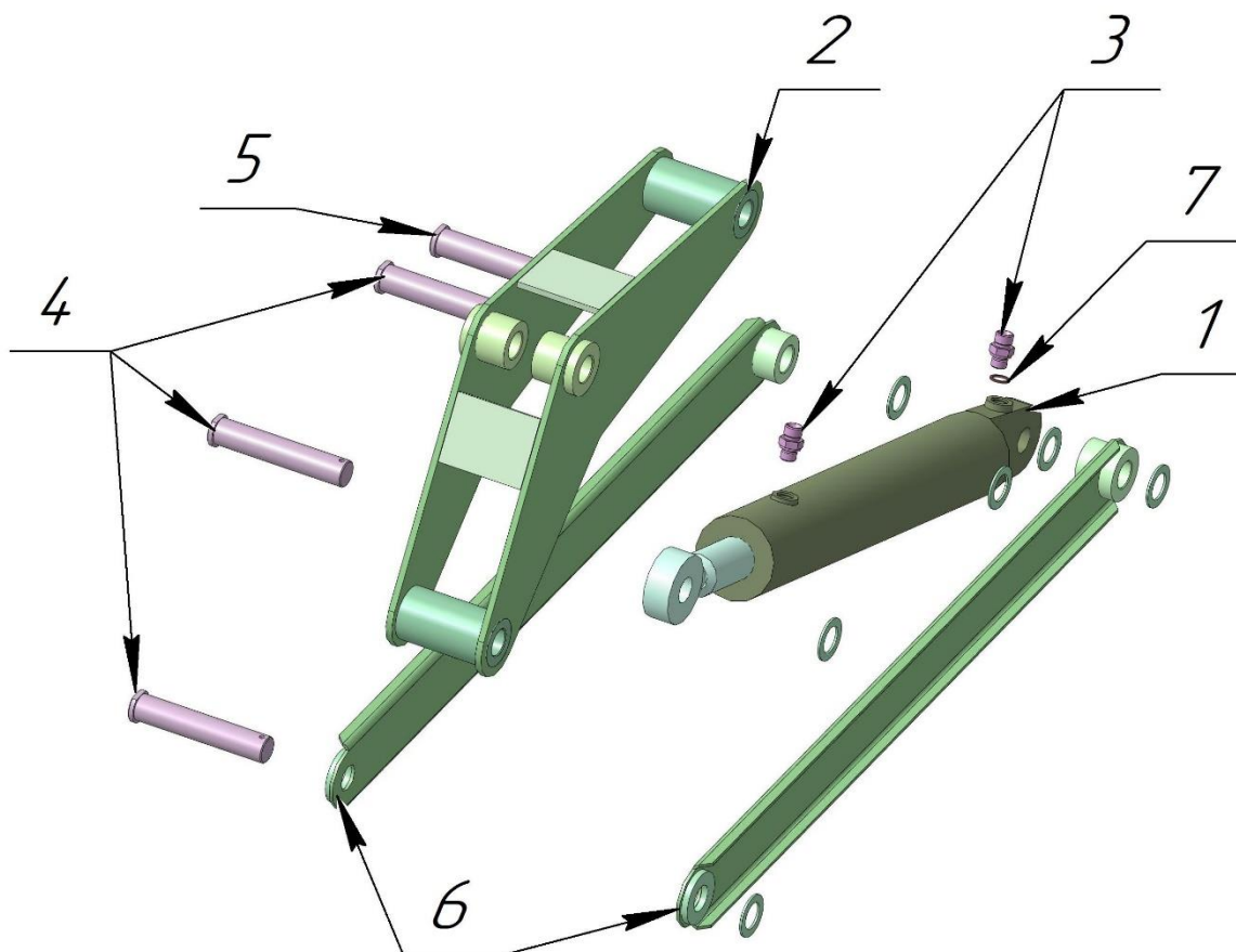
МЕХАНИЗМ ПОДЪЕМА (Рис.9)
