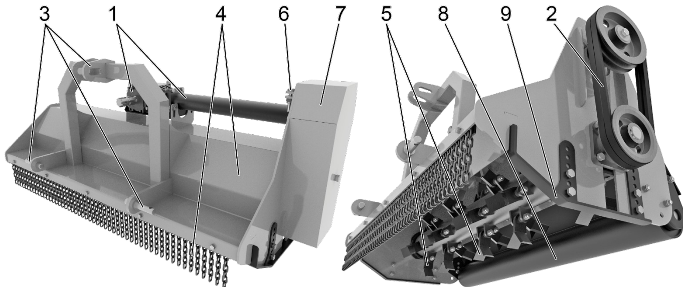
Рис.1 Устройство косилки
