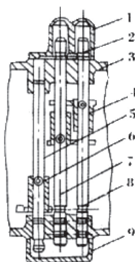
Рис. 3.12. Механизм фиксации передач (для коробки (3x2)+1.
