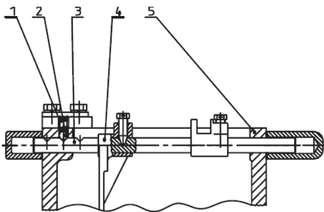
Рис. 3.11. Фиксатор переключения передач.
