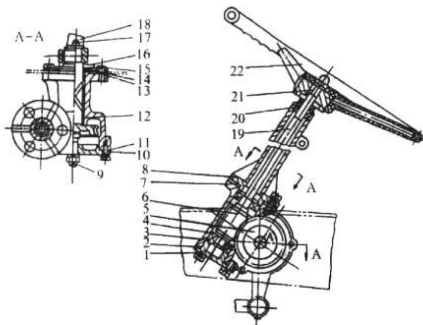
Рис. 3.14. Рулевое управление.
