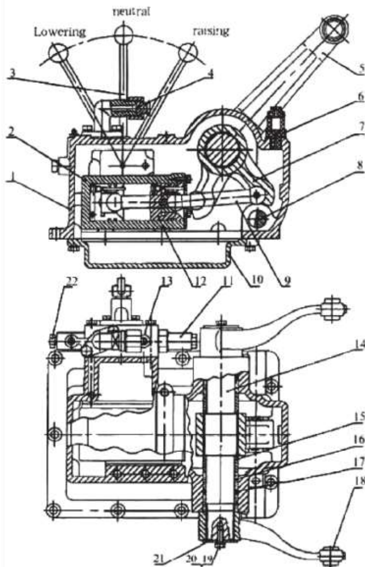
Рис. 3.35. Подъемник.
