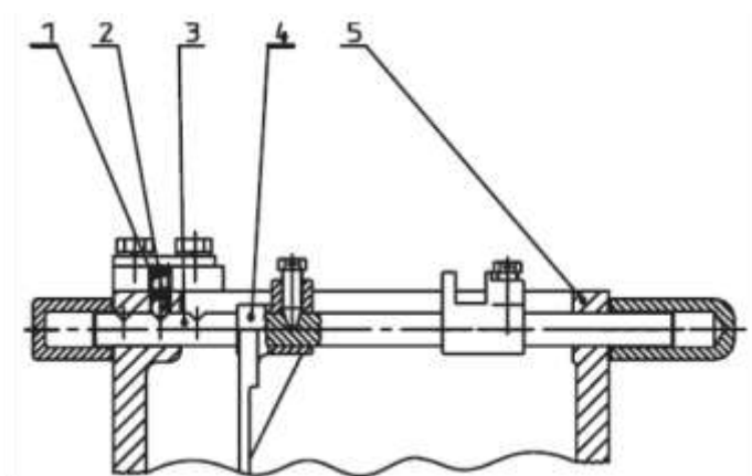
Рис. 3.11. Блокировочный механизм.
