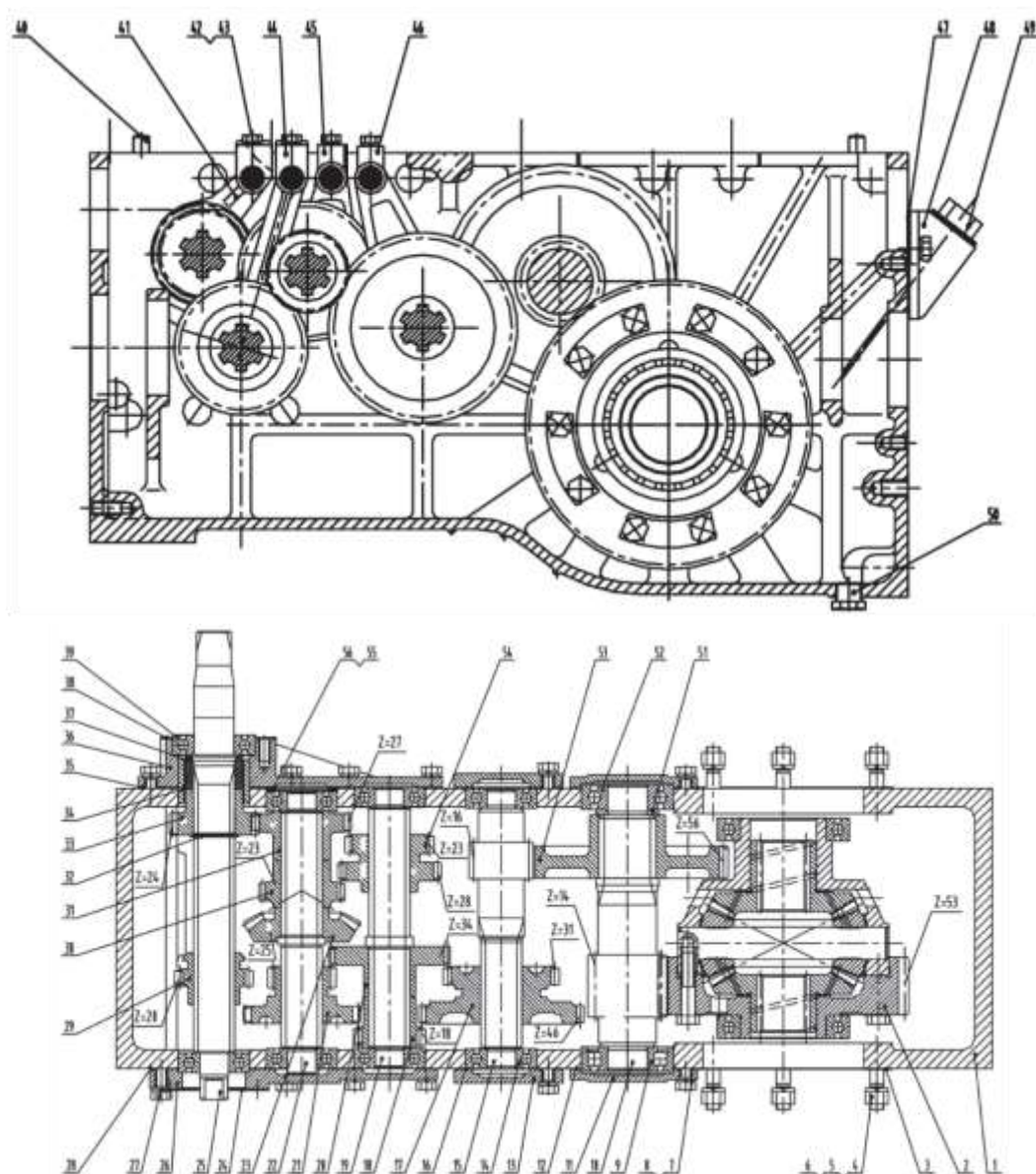
Рис.3.7. Коробка передач (4+1) × 2с отбором мощности, оснащенная шестеренчатым насосом.
