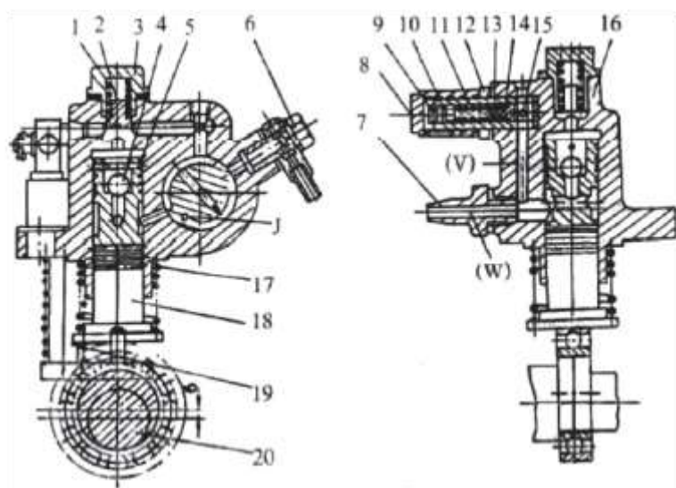
Рис. 3.26. Поршневой насос.
