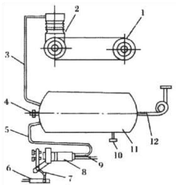
Рис. 3.18. Структура пневмотормоза.
